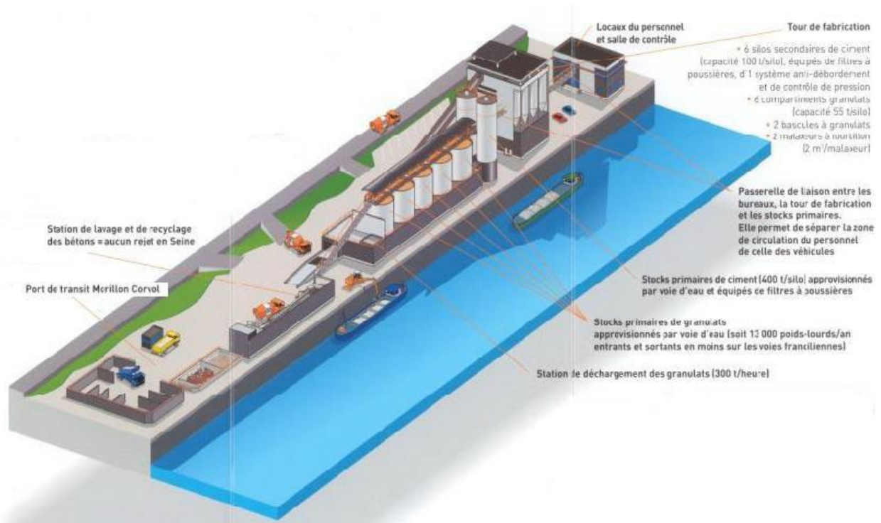
Figure 1 : description d'un site de centrale BPE
