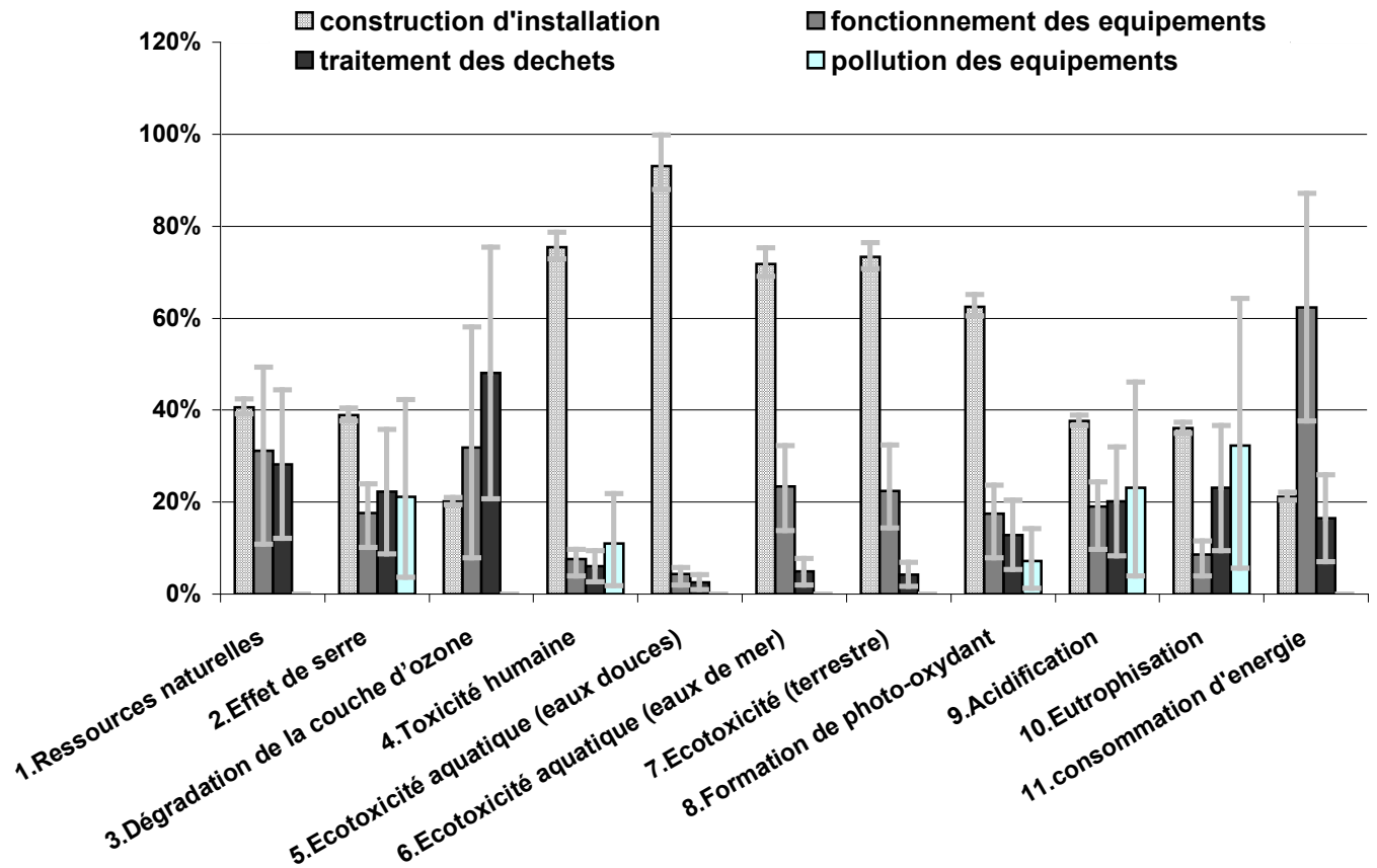
Figure 2 : Contributions relatives de différents aspects du système 'centrale BPE' pour la production de 1m 3 de béton avec leurs variations d'après Chen (2009).
