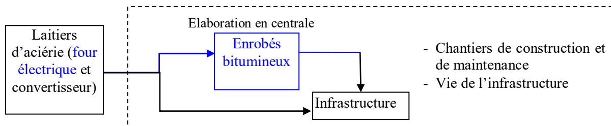
Figure 2: Système d'utilisation des laitiers d'aciérie
