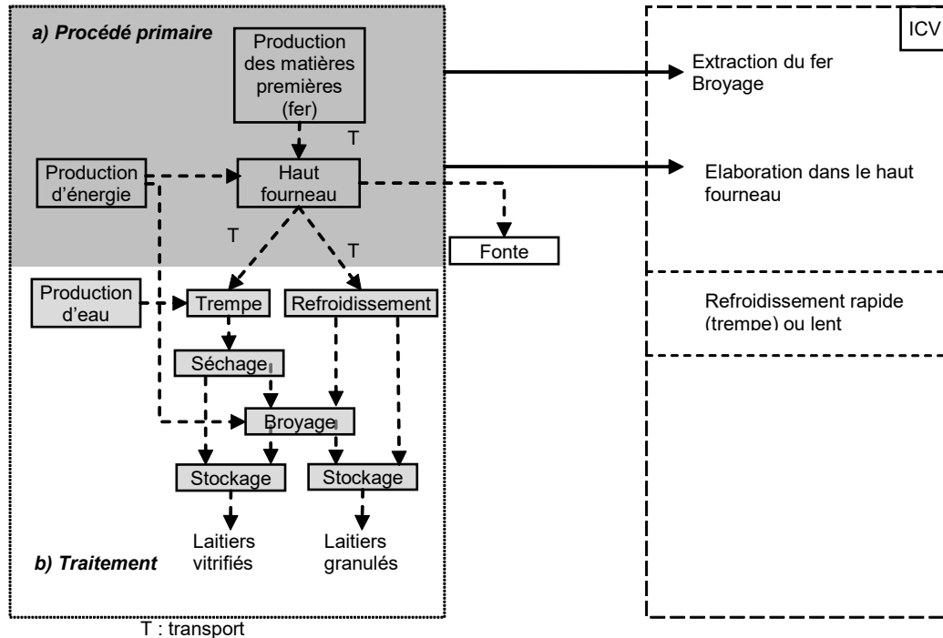
Figure 1 : Système de production primaire, d'après Chen, 2009.
